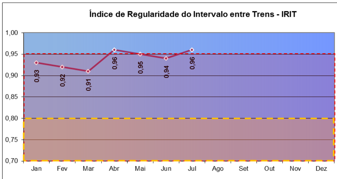
Gráfico 3-17 Metrô – IRIT
