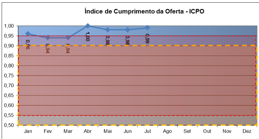
Gráfico 3-16 Metrô – ICPO
